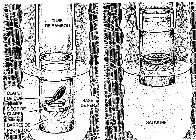
5. LA SAUMURE était remontée du fond du puits à l'aide de tubes de bambou. Un clapet installé sur la partie inférieure du tube s'ouvrait lorsque le tube était plongé dans la saumure, et se refermait lorsque le tube était remonté.
